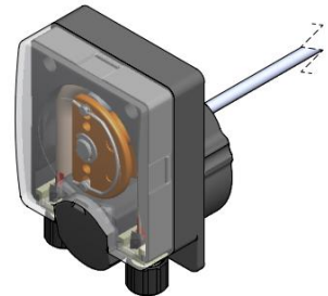
SLIM Line DSP1501-OR 24V Item number: 1002970
